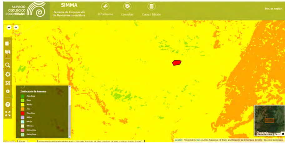
Figura 10. Zonificación de amenaza por movimientos en masa (SGC).
